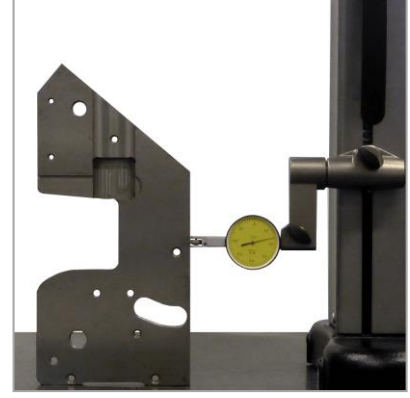
Mesure de perpendicularité avec comparateur à levier ou palpeur électronique
