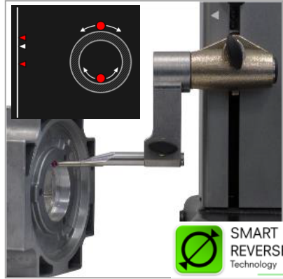
SMART REVERSE: Mesures de diamètres plus simples, plus rapides et plus précises
