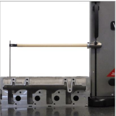
Touches jusqu'à 400 mm avec excellente répétabilité
